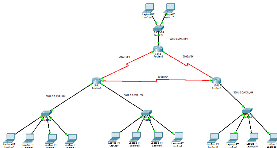
Figura 5: Enrutamiento dinámico
